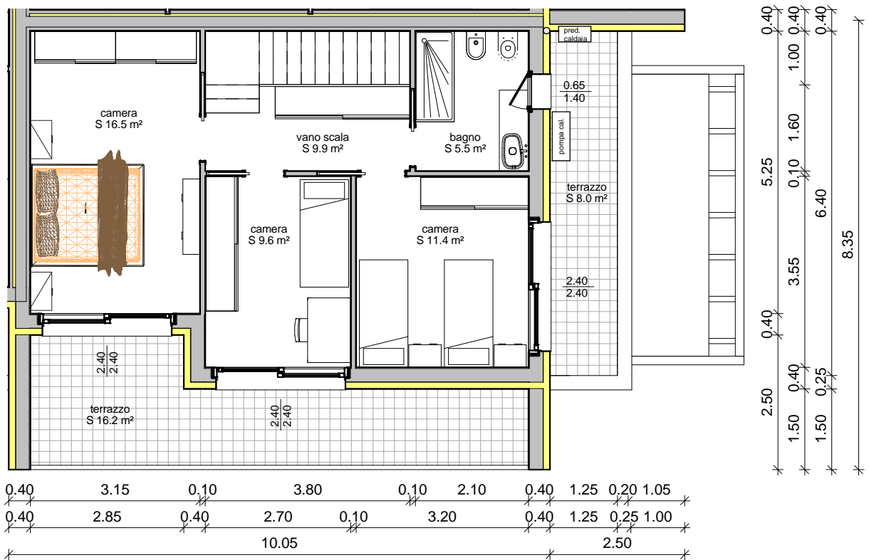
Piano primo
